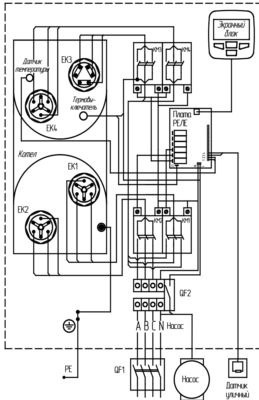
Рисунок 5. Схема подключения ЭВАН UNIVERSAL -36 - 11 -
